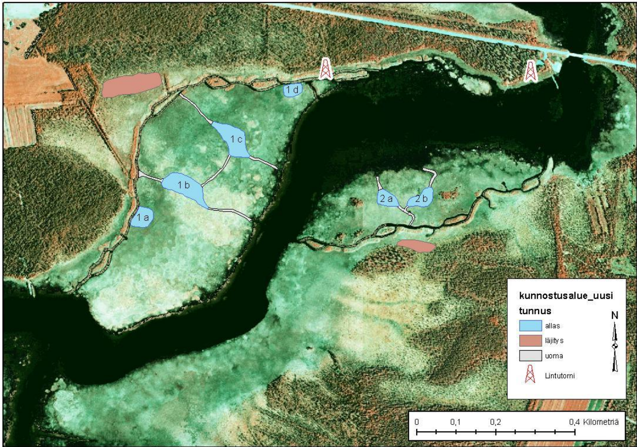
Kuva 2: Juntusjärven luhta-aluekunnostuksen kohteet v. 2012-2013
